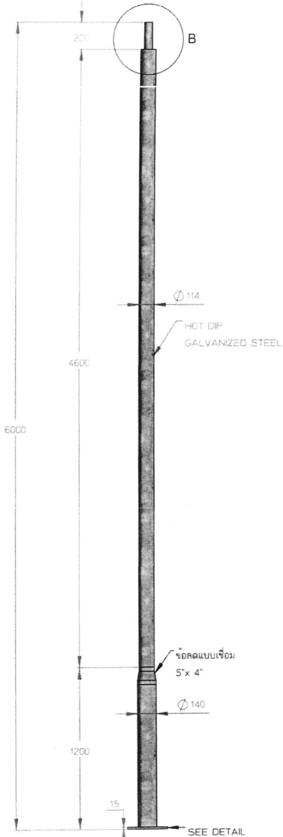
SEE DETAIL BASE PLATE HI-WC5-060:เสาทอมสูง6เมตรขนาด5นิ้วลด4นิ้ว SCALE 1 : 28
